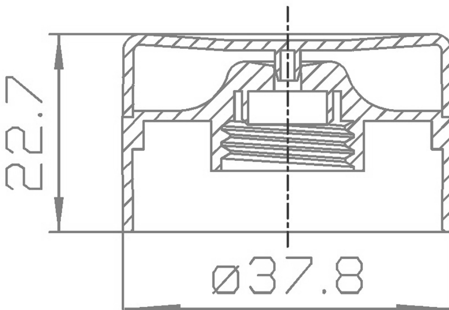
Aggancio a vite/ screw on/ à vis
